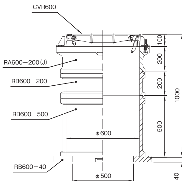
レジンコンクリート組図例 土被り1200mm (CVR600)
