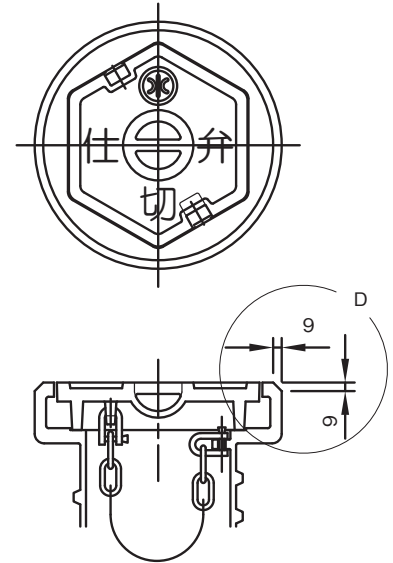
除雪車対応型 (AHE155S)
