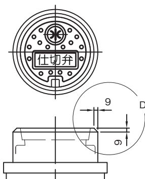
除雪車対応型 (HVB200S)
