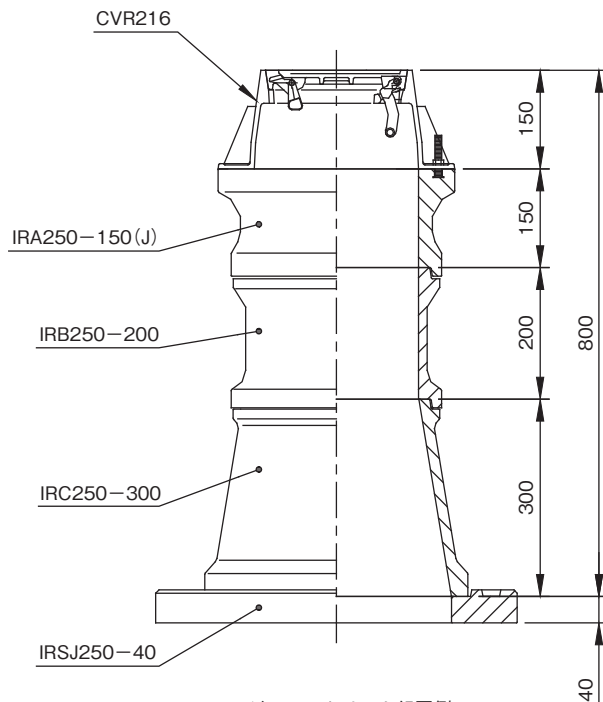
レジンコンクリート組図例
