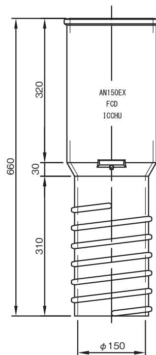
AN150EX 延長継手
