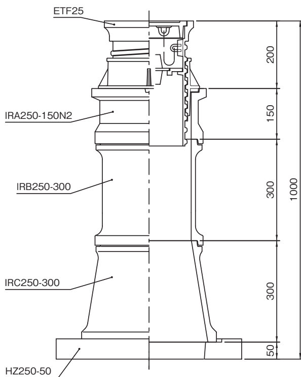
レジコンクリート組図例 土被り1200mm
